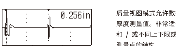
实时A-Scan，用于更精密地评估
