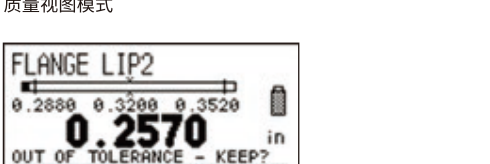
超差对话框
