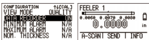
选择质量视图模式显示屏
